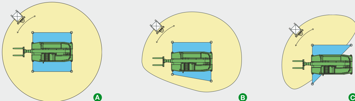
Die Maschine bei einer unkonventionellen Geometrie der Aufstützfläche auf dem Boden voll einsatzfähig zu machen ist mit dem System MCSS möglich: gleich welches Polygon der Standsicherheit vorliegt, erstellt das System dynamisch eine „virtuelle“ Arbeitskurve, innerhalb derer die volle Einsatzbarkeit der Maschine und die volle Ausnutzung des maximalen für die gegebene Konfiguration erzielbaren Lastdiagramms garantiert ist, gleich welches Anbaugerät verwendet wird, einschließlich Hubarbeitsbühnen. Bei maximal ausgefahrenen Abstützungen (Abb. A) ist für den Arbeitsbereich während der gesamten Drehung des Oberwagens der volle Einsatz gesichert. Der Arbeitsbereich wird automatisch vom Bordcomputer begrenzt, wenn die Geometrie der Aufstützfläche gemäß der Arbeitsanforderungen konfiguriert ist, z.B. bei einer nur teilweise ausgefahrenen Abstützung (Abb. B). Eine Grenzsituation tritt ein, wenn eine der Abstützungen den Boden nicht berührt, z.B. aufgrund des Nachgebens der Aufstützfläche (Abb. C). Auch in diesem Fall wird der Arbeitsbereich automatisch begrenzt.
